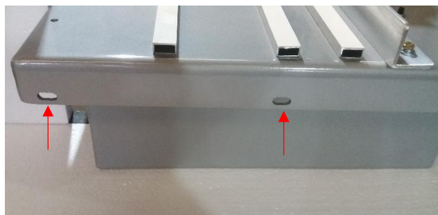
Figura 7 - Pontos de fixação
