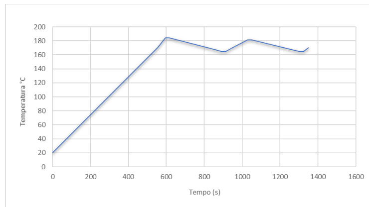
Figura 10 - Comportamento da temperatura do coleiro
