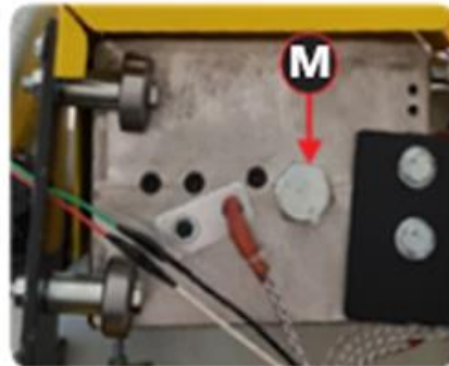
Figura 16 - Bujão de escoamento
